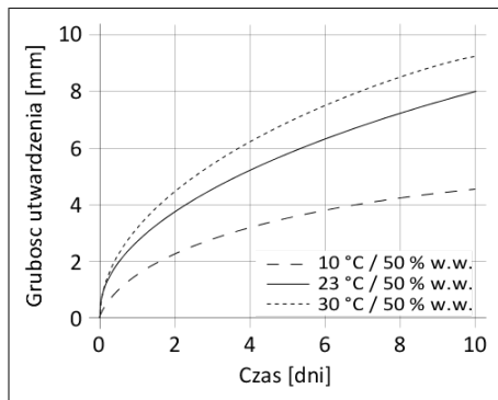
Wykres 1: Szybkość utwardzania Sikaflex®-591
